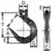
22013VWH... Gancho boca ancha
